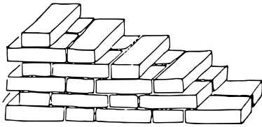
5) Gotischer Verband
