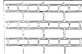
20) Schichtenmauerwerk (opus mixtum) Beisp.: Quader- und Ziegelsteine
