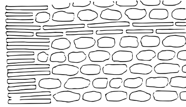
1) Feldsteinmauerwerk, Beisp. mit Eckverquaderung und Ausgleichschichten
