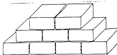
13) Quadermauerwerk, Quader gleichgroß, gleichhohe Schichten (opus isidomum)
