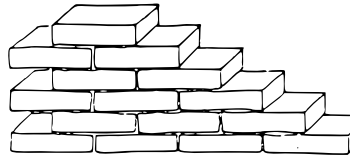
1) Läuferverband
