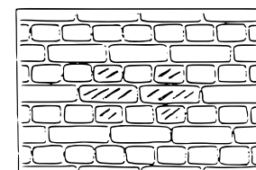
4) Kreuzverband
