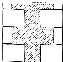
23) Zweischalige Mauer mit Gußkern
