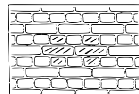
4) Kreuzverband
