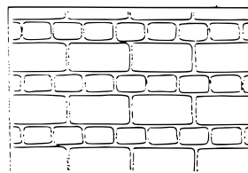
20) Schichtenmauerwerk (opus mixtum) Beisp.: Quader- und Ziegelsteine
