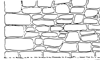
2) Bruchsteinmauerwerk (opus antiquum) mit Eckverquaderung
